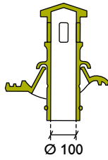
doorvoerpan (met doorvoer voor dakhelling 25° - 45°)
