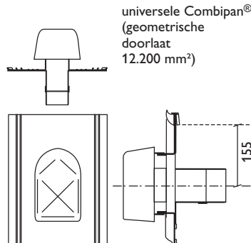
aansluitpan
