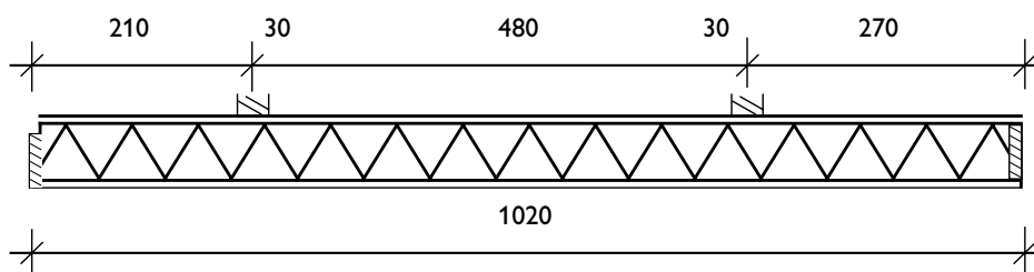
Dwarsdoorsnede sandwich-dakelement met zijribben
