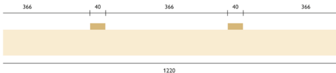
Doorsnede CBRP element
