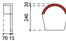
uni-begin-/eind afdekkap
