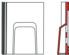
ventilatiepan (ventilatieopening ca. 2.500 mm 2 )
