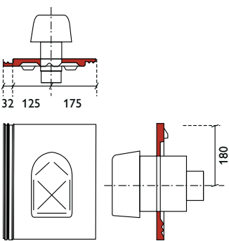
combipan Stonewold (geometrische doorlaat 12.200 mm 2 )
