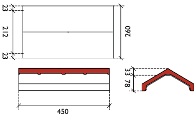
hoekige vorst
