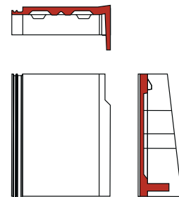
ondergevelpan rechts
