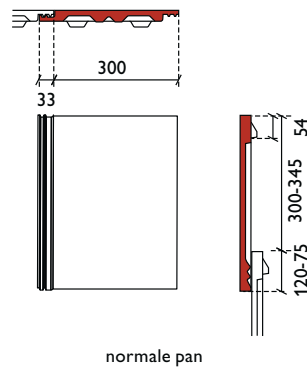
normale pan
