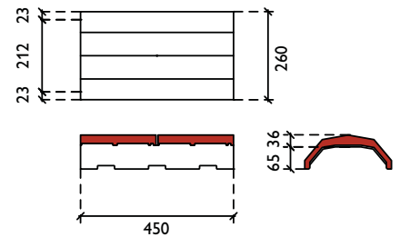
HV vorst
