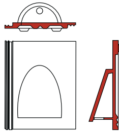
huismussenpan
