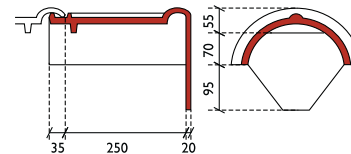
halfronde beginvorst model Tegelen
