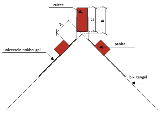
nokbeugel geknikt op perforatie
