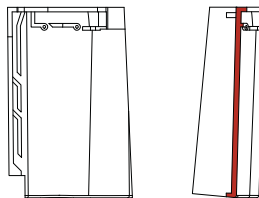
ondergevelpan rechts
