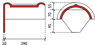
halfronde eindvorst model Tegelen
