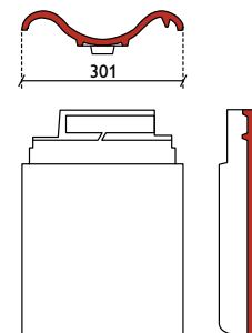
dubbele welpan
