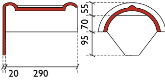
halfronde eindvorst model Tegelen
