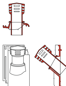
doorvoerpan + ventilatiekoker (met doorvoer voor dakhelling 25° – 45°)
