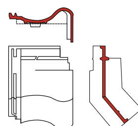
knikgevelpan rechts 140°
