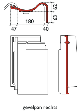
gevelpan rechts
