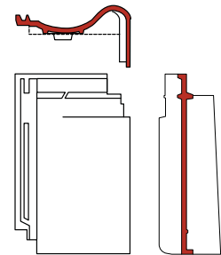
ondergevelpan rechts
