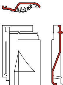
ventilatiepan (ventilatie-opening 500 mm 2 )
