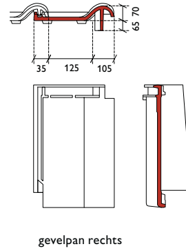
gevelpan rechts
