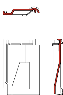
ventilatiepan (ventilatie opening ca 2.000 mm 2 )
