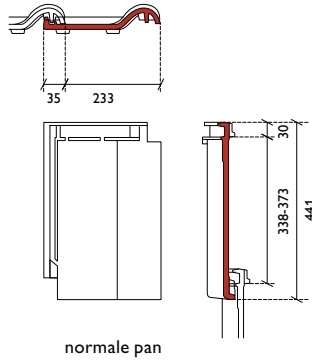
normale pan
