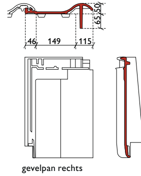
gevelpan rechts
