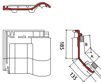
knikpan
