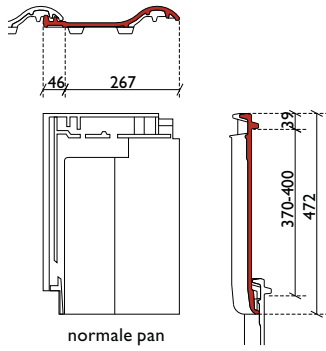
normale pan
