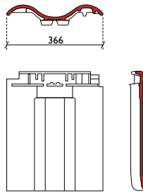
dubbele welpan
