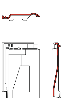
ventilatiepan (ventilatie opening ca 2.000 mm 2 )
