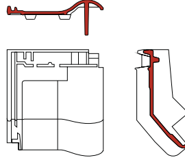
knikgevelpan rechts
